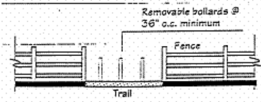
A: Elevation -- Bollards
