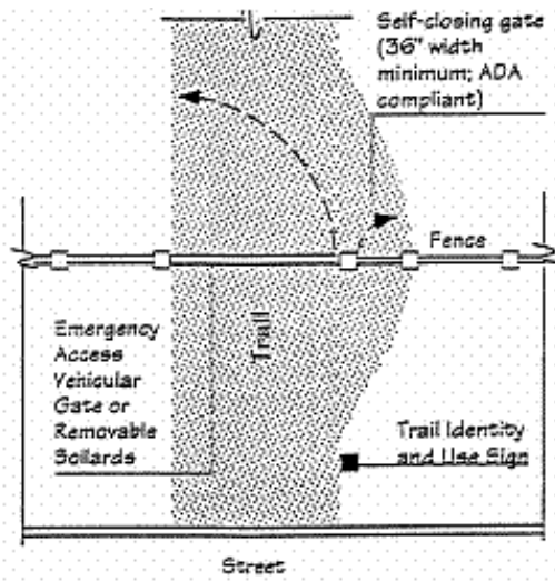
A: Plan -- Trail Gates
