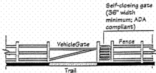
A: Elevation -- Trail Gates
